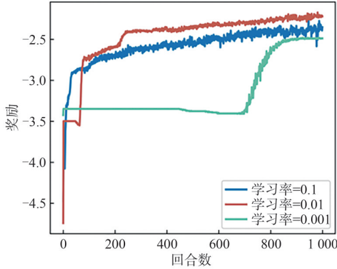
图6 TD3-HAO算法MD任务卸载智能体在不同学习率下的奖励曲线
