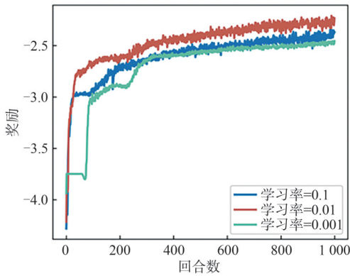
图7 TD3-HAO算法AAN资源分配智能体在不同学习率下的奖励曲线
