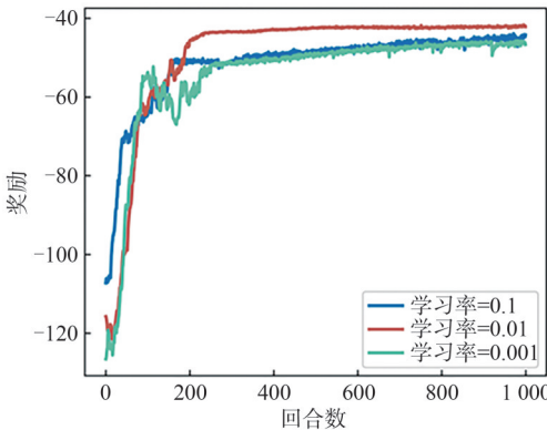
图8 TD3-HAO算法AAN轨迹规划智能体在不同学习率下的奖励曲线
