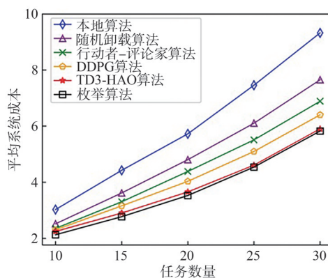
图11 不同任务数量下TD3-HAO算法与基准算法的平均系统成本对比
