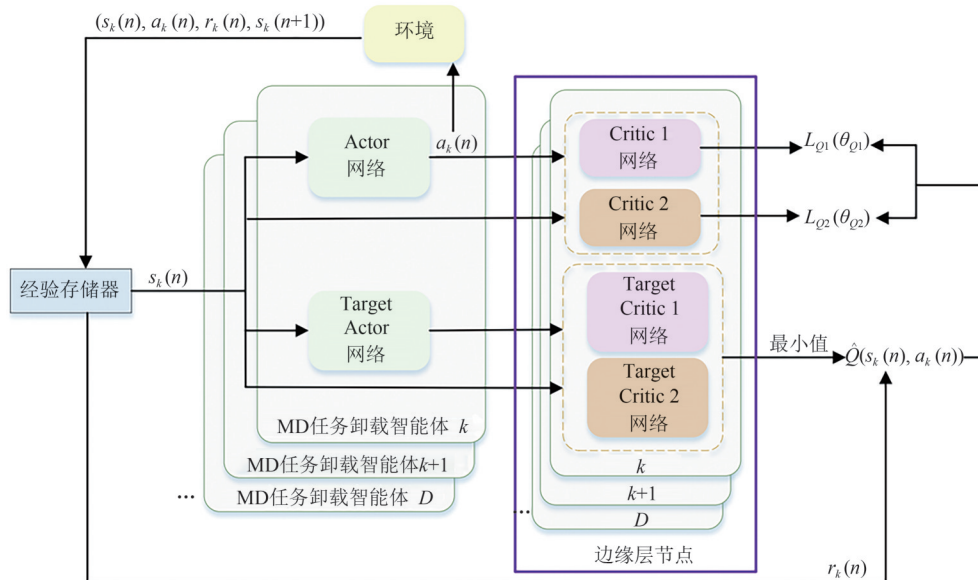
图4 TD3网络结构及工作流程
