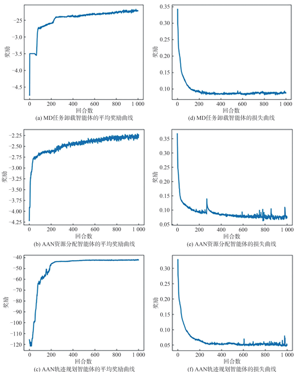
图 5 TD3-HAO 算法各智能体的平均奖励曲线和损失曲线
