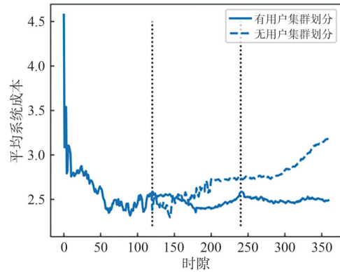
图9 用户集群划分算法对平均系统成本的影响
