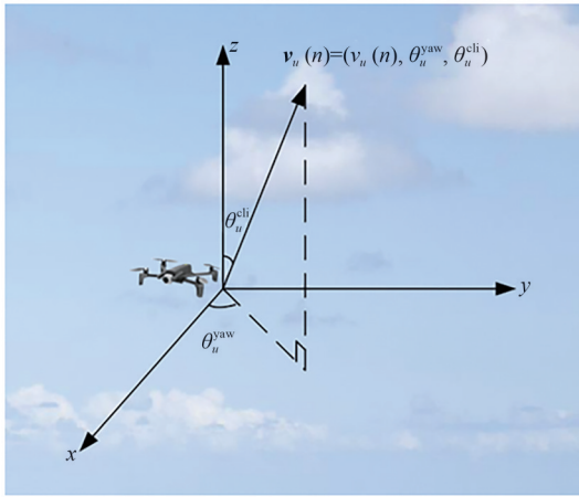
图2 空中节点移动示意
