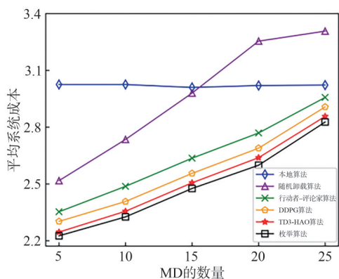
图10 不同MD数量下TD3-HAO算法与基准算法的平均系统成本对比
